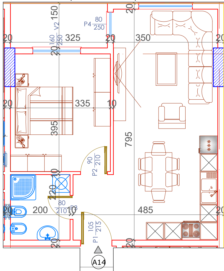
PLANIMETRIA E APARTAMENTIT NR 14 KATI TIP (KATI TRETË +11.34) SH.1:75
