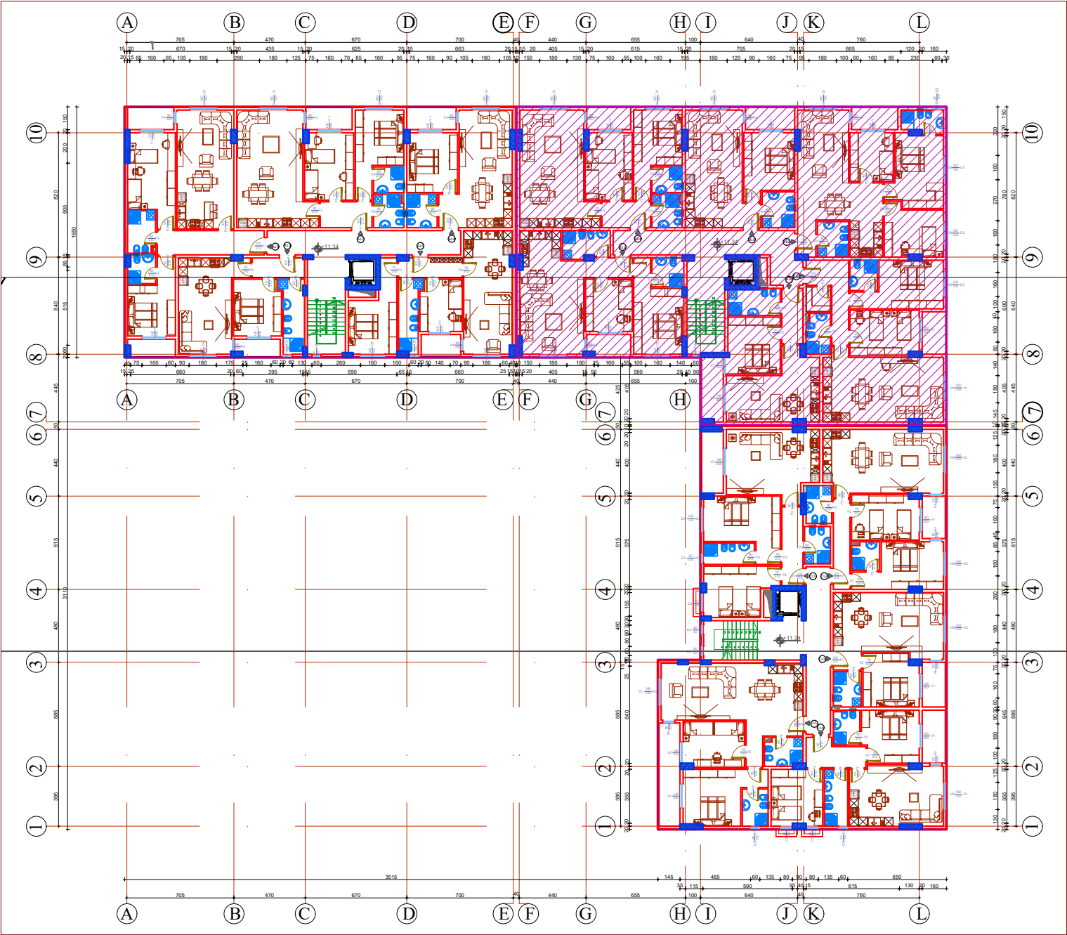
PLANIMETRIA E KATIT TIP (KATI TRETË +11.34) , SEKSIONI A SH 1:350
