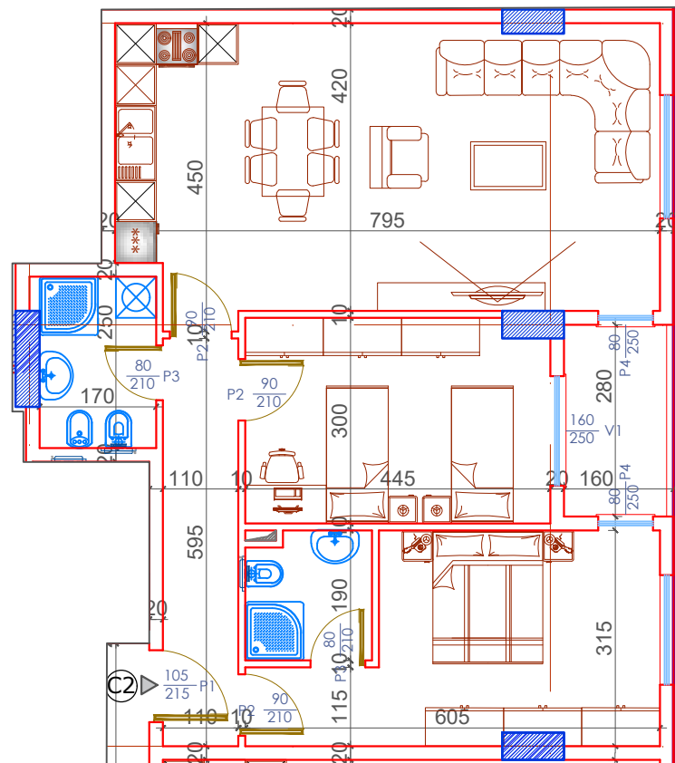
PLANIMETRIA E APARTAMENTIT NR 2 KATI TIP (KATI PARË +5.04) SEKSIONI C
