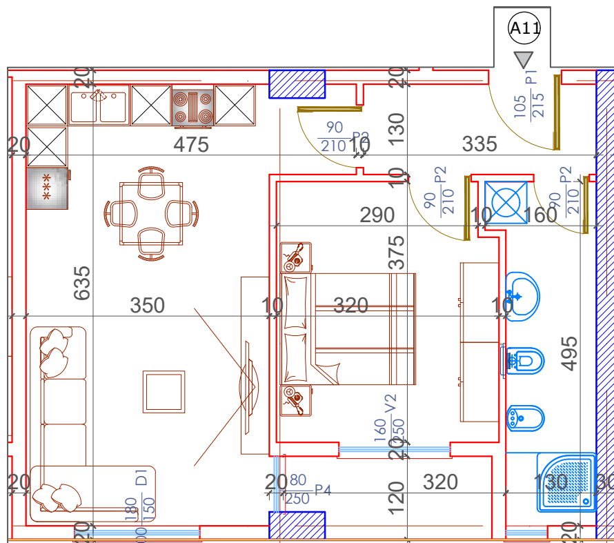
PLANIMETRIA E APARTAMENTIT NR 11 KATI TIP (KATI TRETË +11.34) SH.1:75
