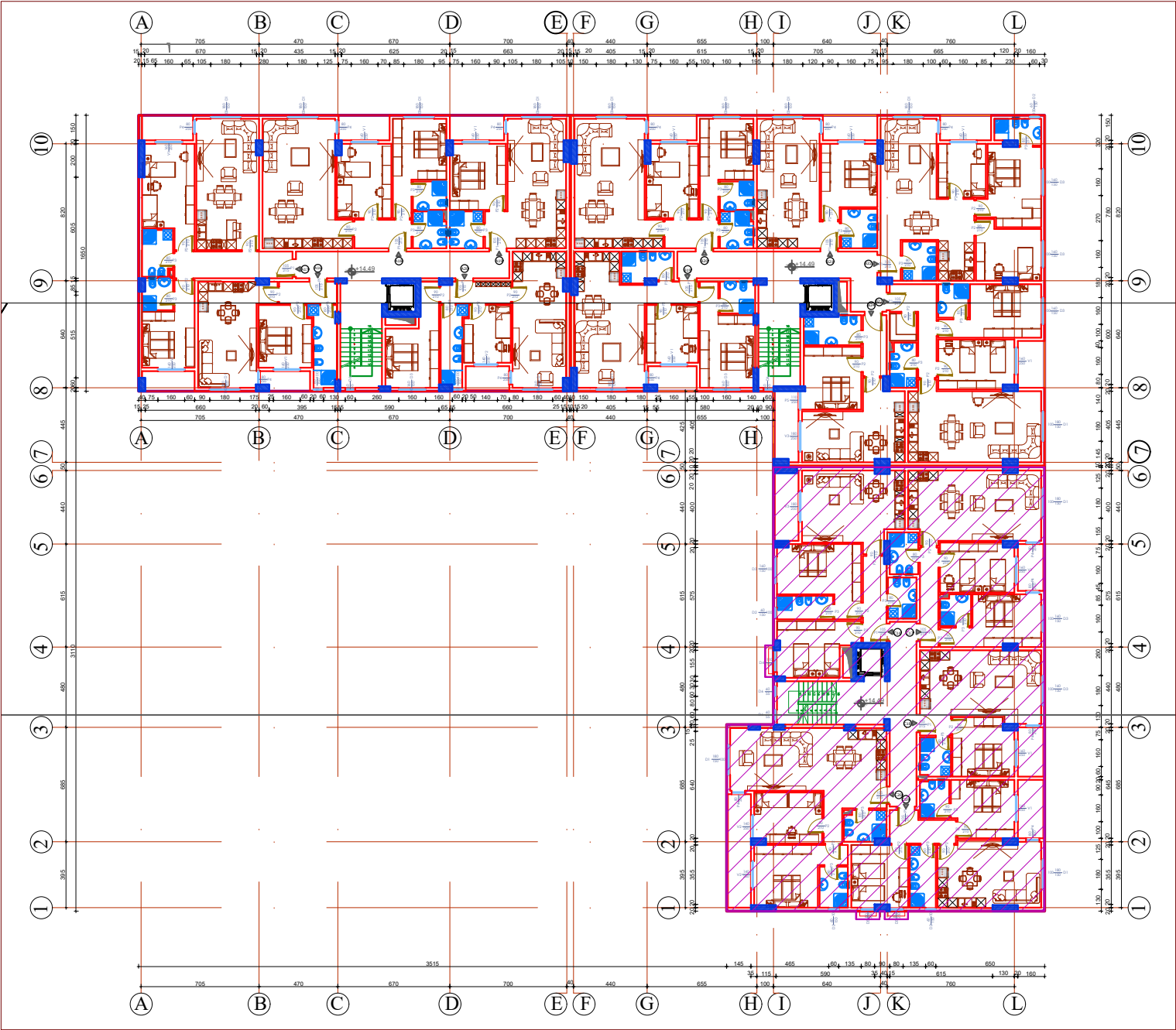
PLANIMETRIA E KATIT TIP (KATI KATËRT +14.49) , SEKSIONI C SH 1:350
