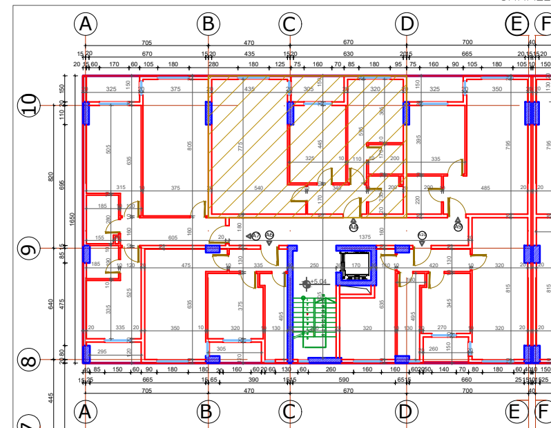
KATI DYTË
