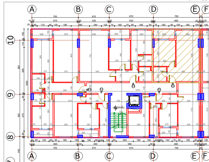
KATI PARË
