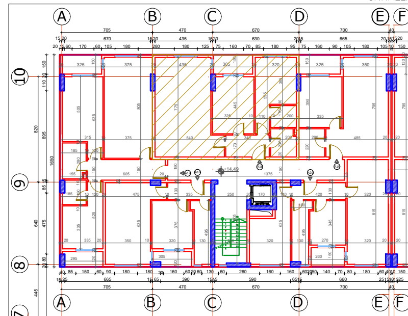
KATI KATËRT
