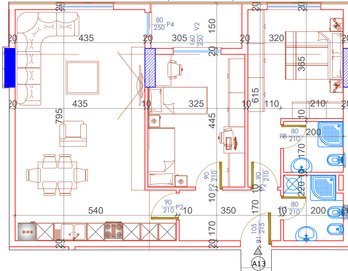
PLANIMETRIA E APARTAMENTIT NR 13 KATI TIP (KATI TRETË +11.34) SH.1:75
