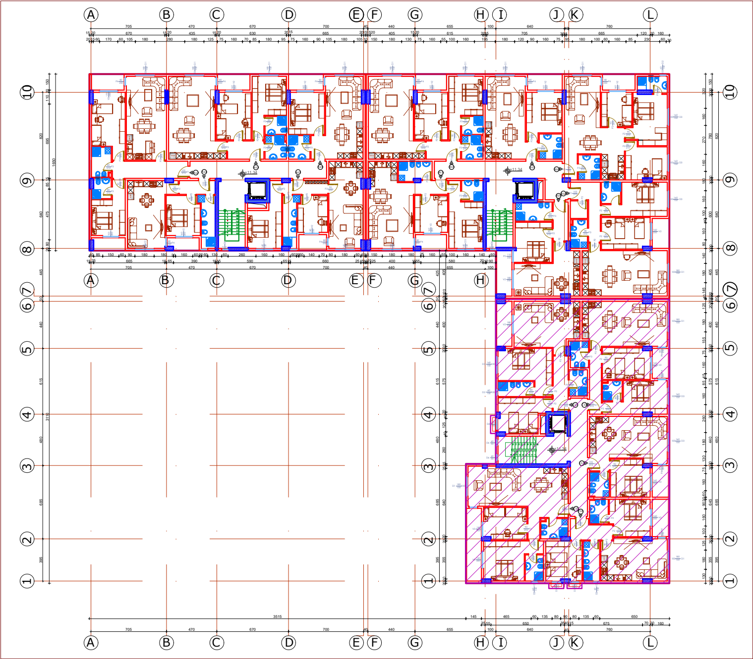
PLANIMETRIA E KATIT TIP (KATI TRETË +11.34) , SEKSIONI C SH 1:350
