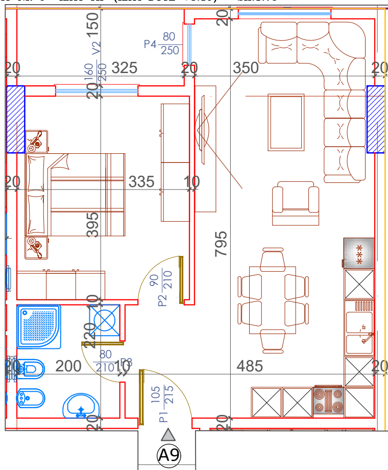
PLANIMETRIA E APARTAMENTIT NR 9 KATI TIP (KATI DYTË +8.19) SH.1:75
