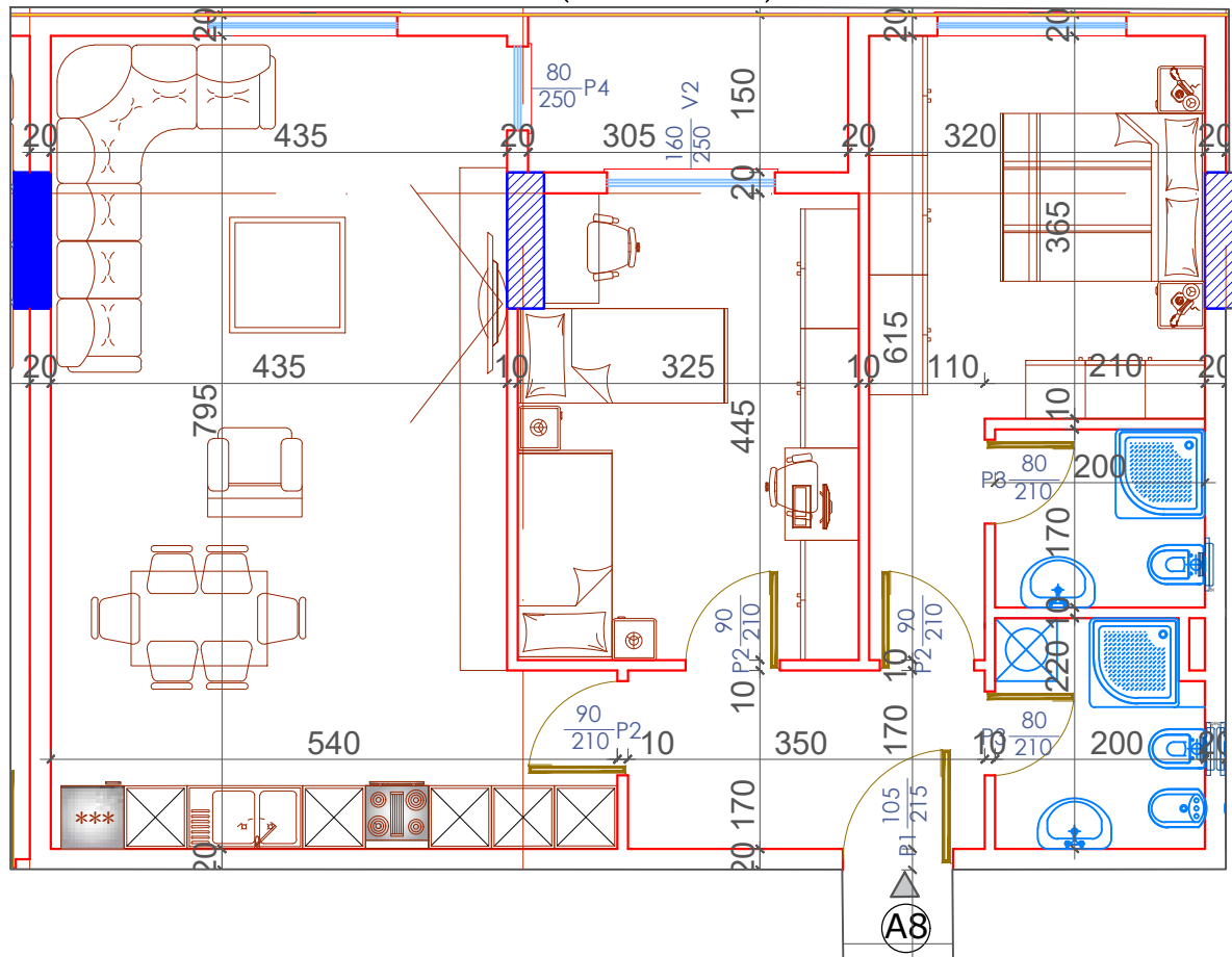
PLANIMETRIA E APARTAMENTIT NR 8 KATI TIP (KATI DYTË +8.19) SH.1:75
