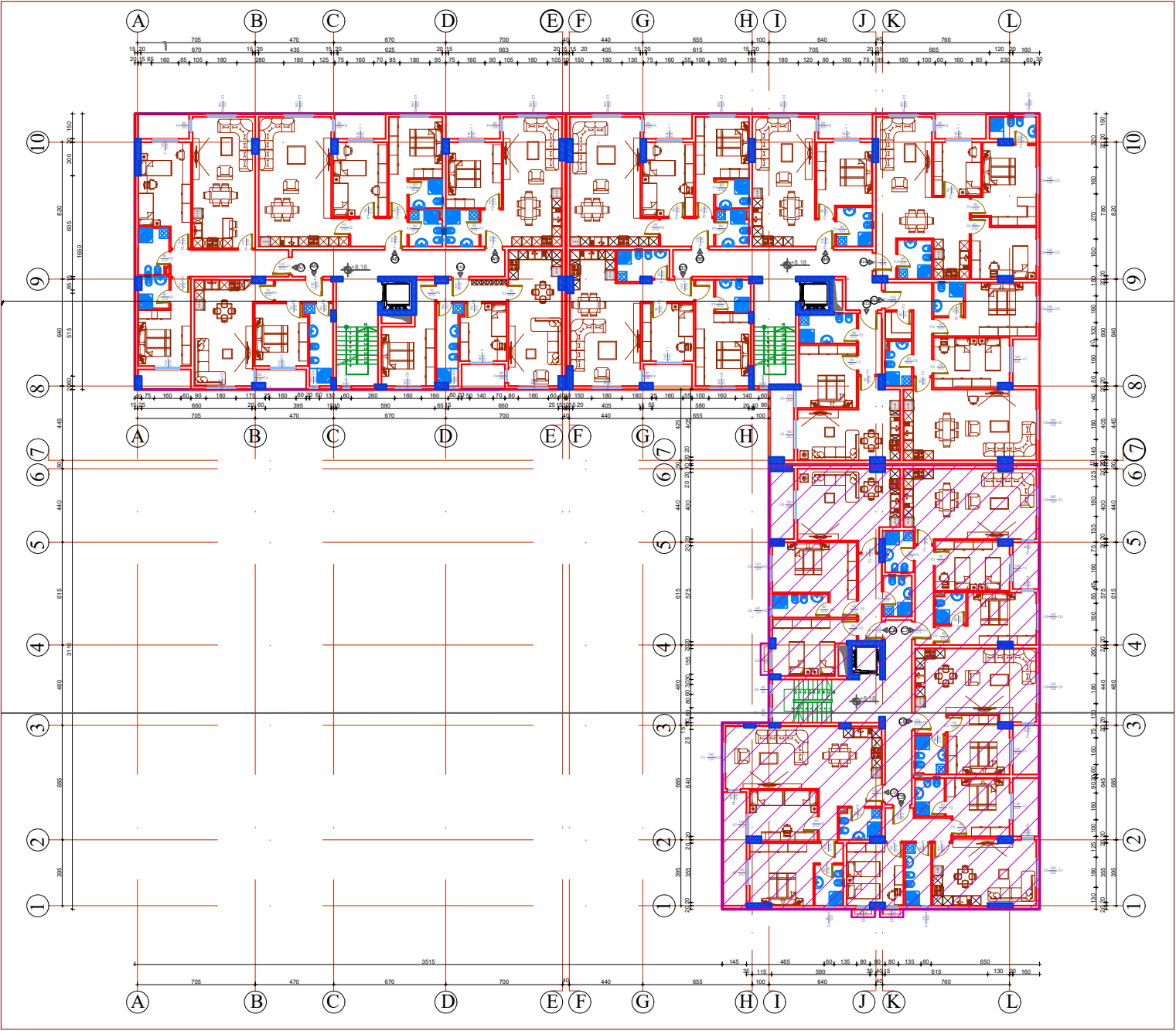
PLANIMETRIA E KATIT TIP (KATI DYTË +8.19) , SEKSIONI C SH 1:350
