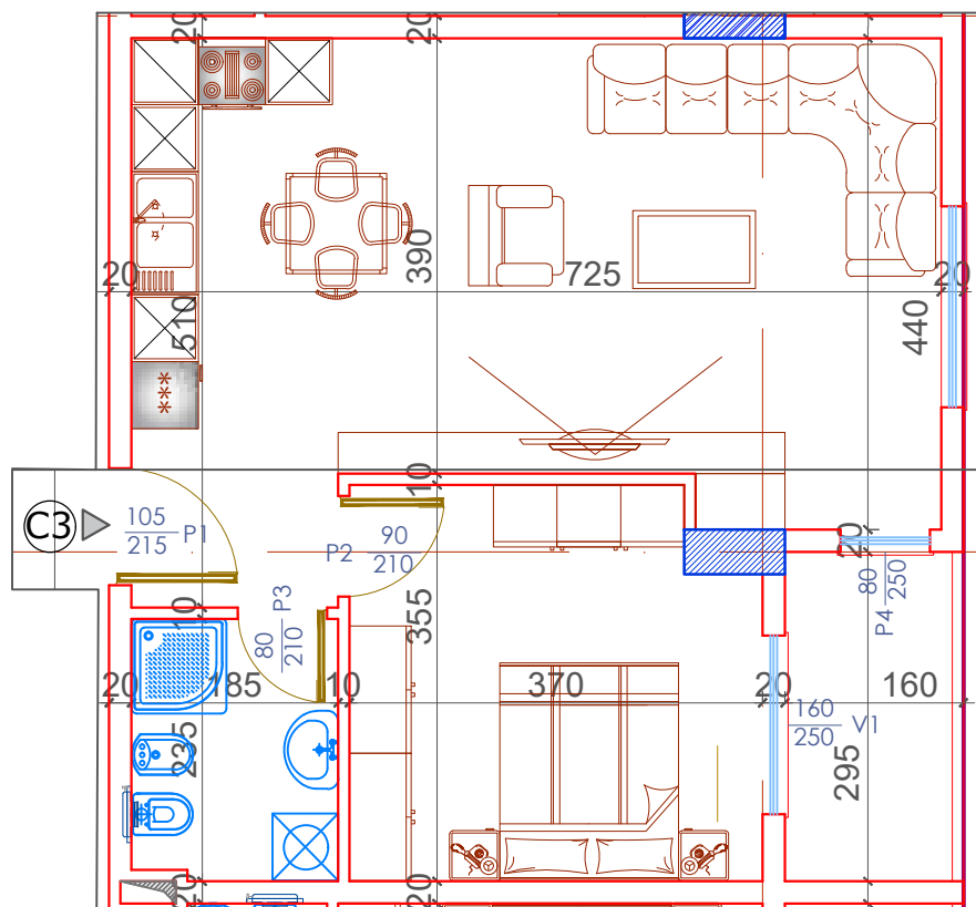
PLANIMETRIA E APARTAMENTIT NR 3 KATI TIP (KATI PARË +5.04) SEKSIONI C SH.1:75
