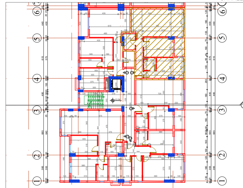
KATI PARĒ SHKALLA 1:350
