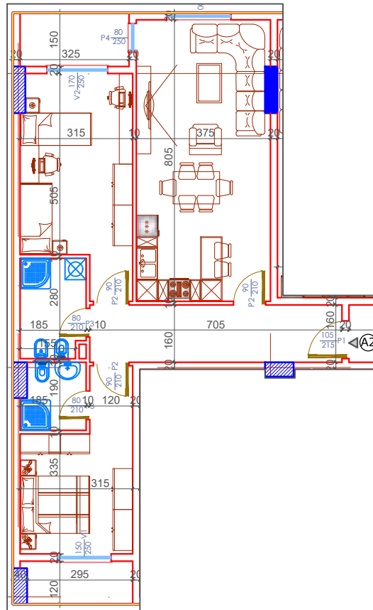
PLANIMETRIA E APARTAMENTIT NR 2 KATI TIP (KATI PARË +5.04) SH.1:150
