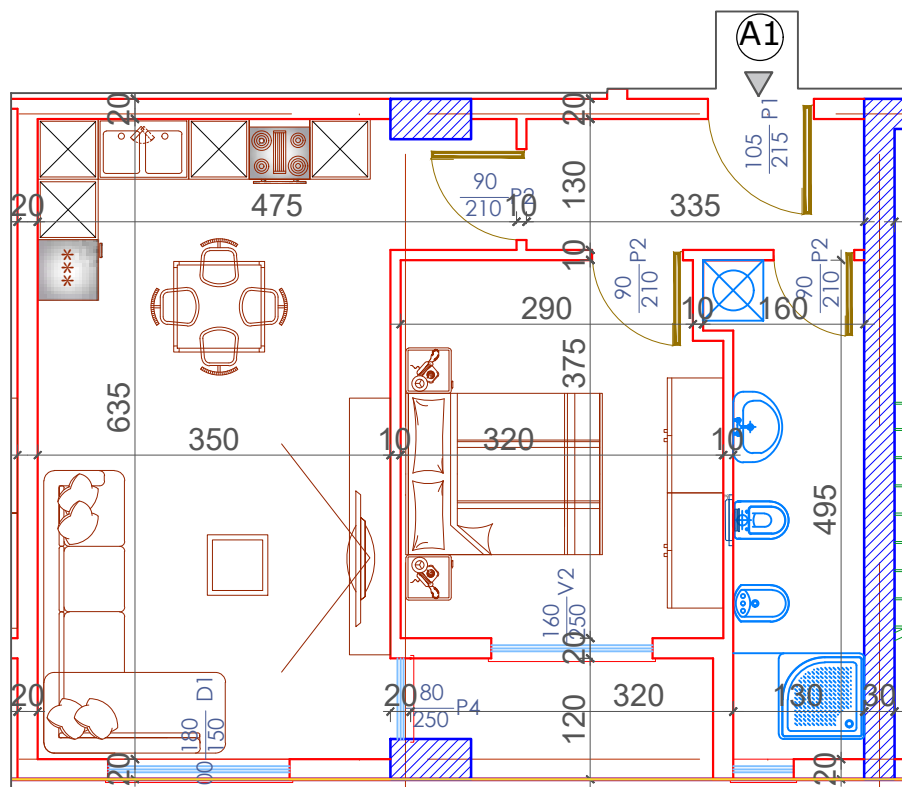
PLANIMETRIA E APARTAMENTIT NR 1 KATI TIP (KATI PARË +5.04) SH.1:75
