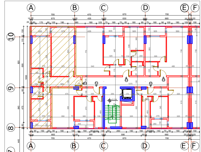
KATI PARĒ SHKALLA 1:300
