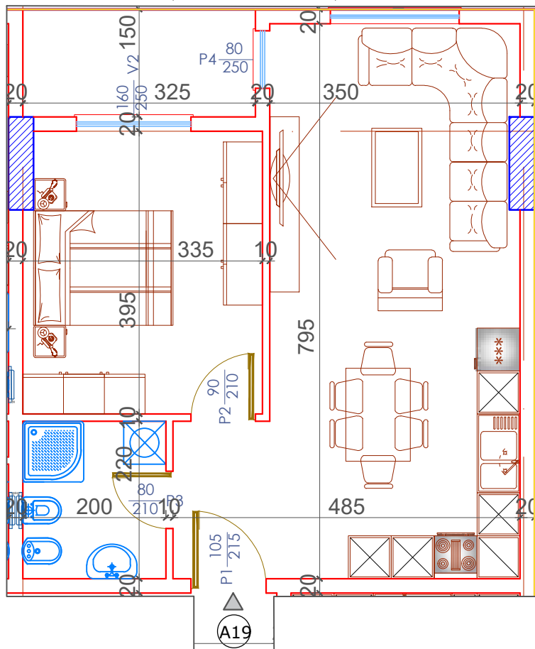
PLANIMETRIA E APARTAMENTIT NR 19 KATI TIP (KATI KATËRT +14.49) SH.1:75
