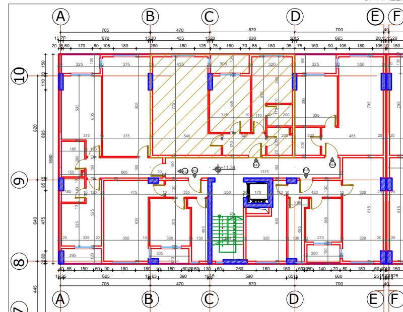
KATI TRETË
