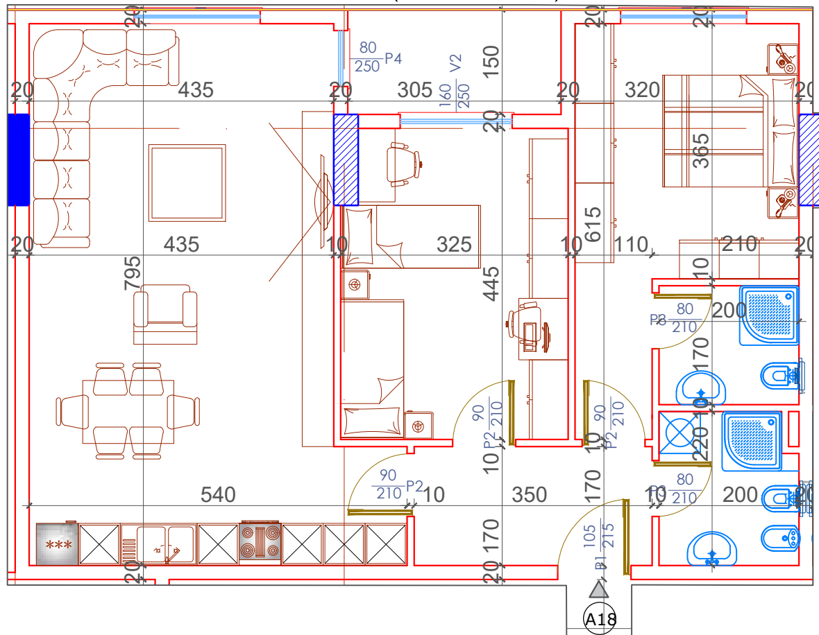
PLANIMETRIA E APARTAMENTIT NR 18 KATI TIP (KATI KATËRT +14.49) SH.1:75
